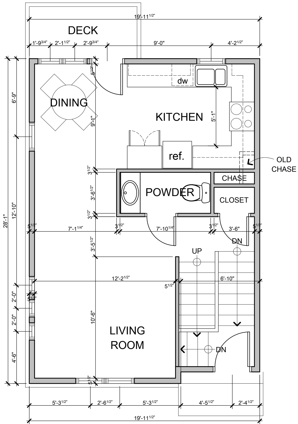
E1 Main Plan
