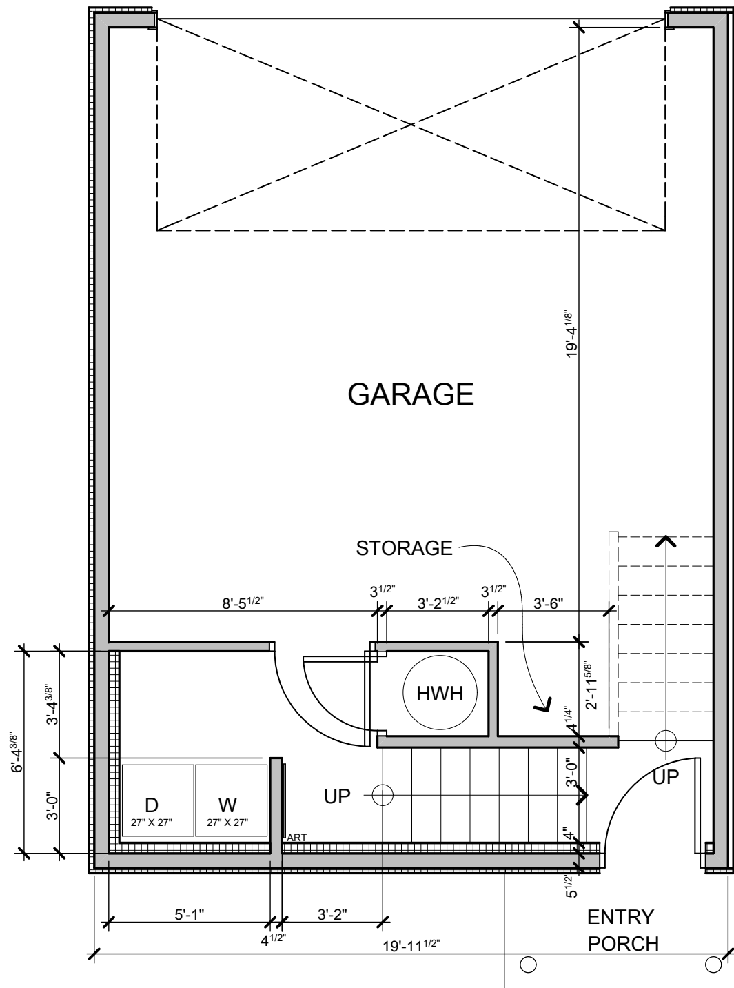
E1 Lower Plan
