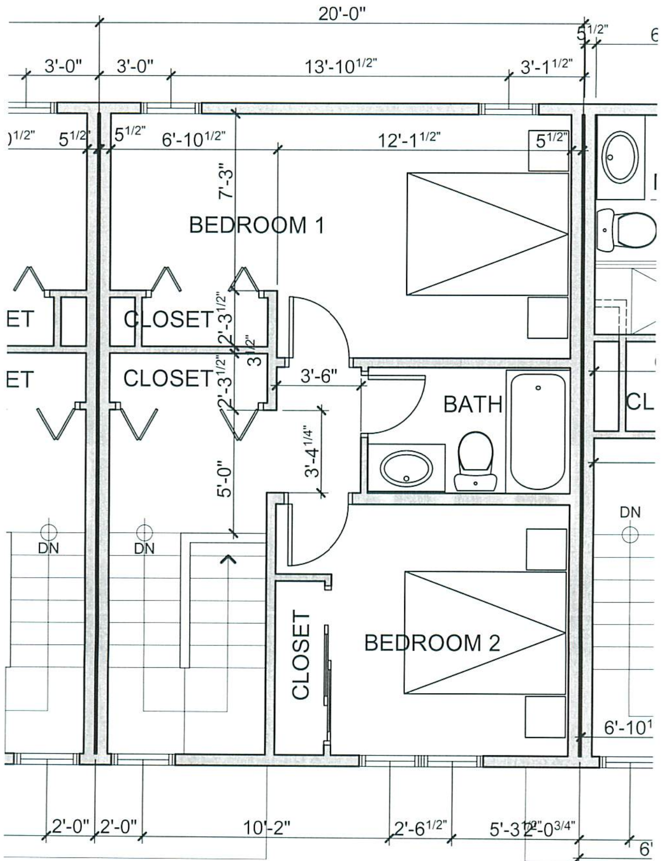
E3 Upper Plan
