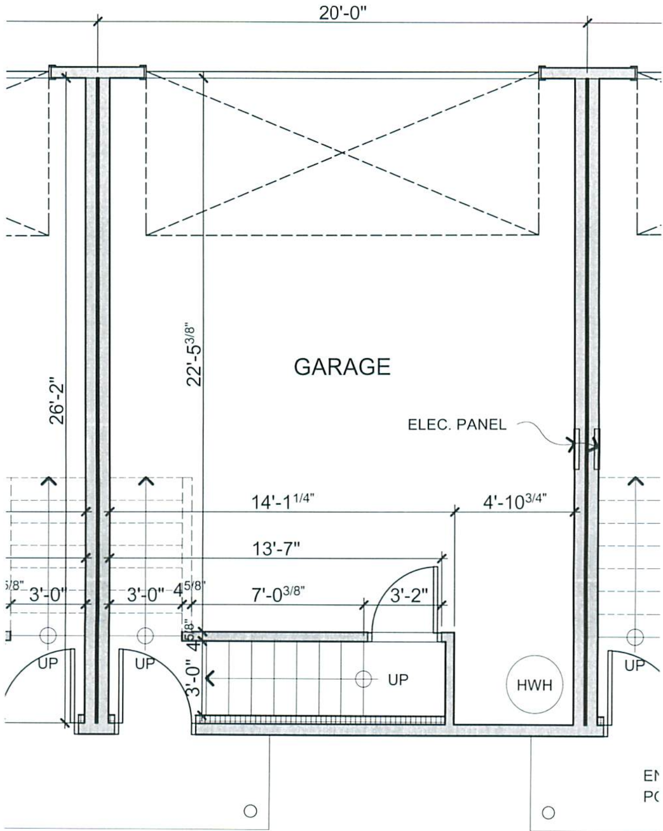
E3 Lower Plan
